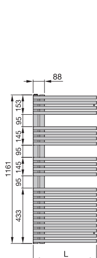
Pohled zepředu, LFAR-120
