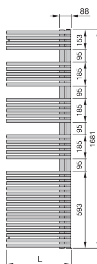
Pohled zepředu, LFAL-170
