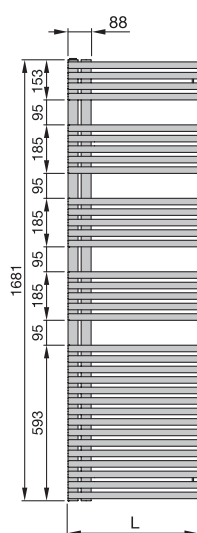
Pohled zepředu, LFAR-170
