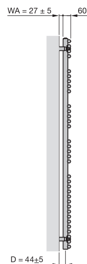
Pohled z boku, LFA(*)-170
